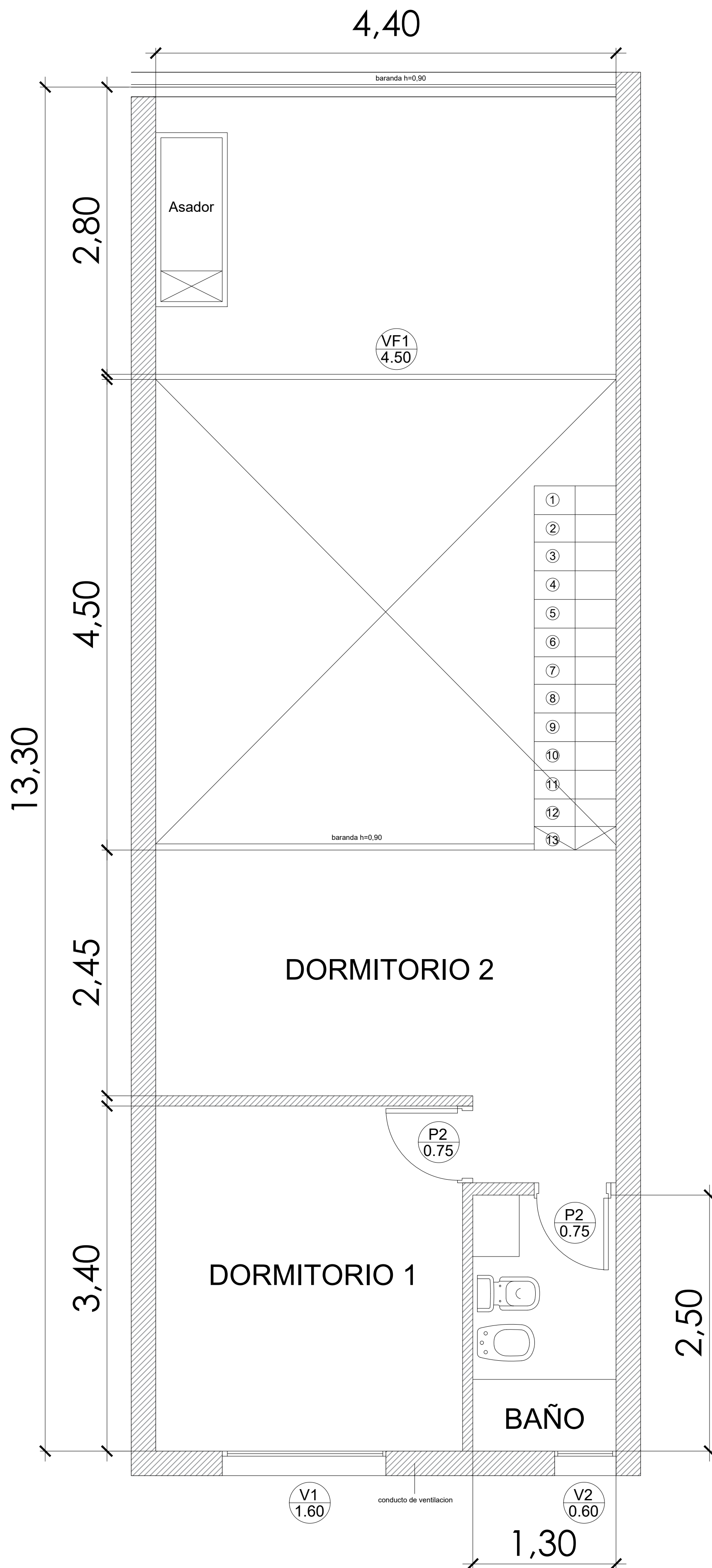
PLANTA ALTA tipologia 2 dormitorios
